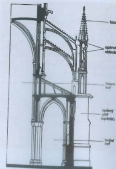
Schéma opěrného systému
